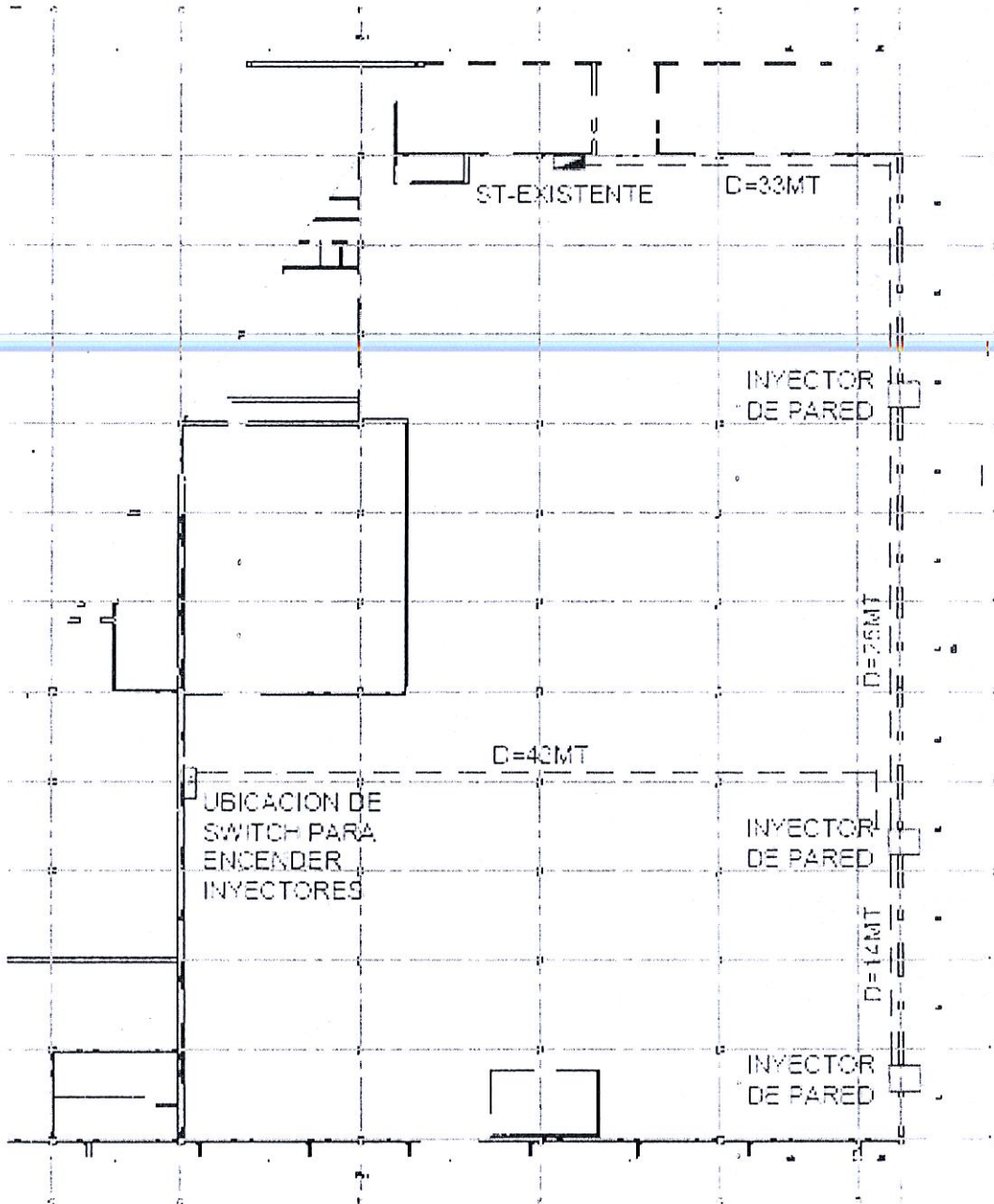
ESQUEMA DE CONEXION DE INYECTORES SALA DE MEDICAMENTOS, ALMACEN SIN ESTERILIZACION EN EL PARANSAZ
